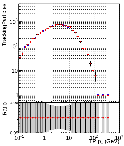
—•— DQM_mkFit_TT_base_noSel —•— DQM_mkFit_TT_retrainOldFiles_v2_8iter2_noSel
