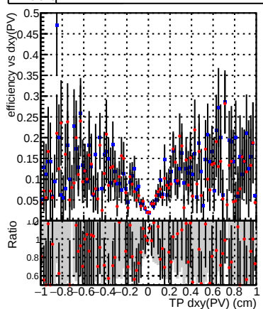
Efficienc — DQM_mkFit_TT_retrainOldFiles_v2_8iter2_noSel
