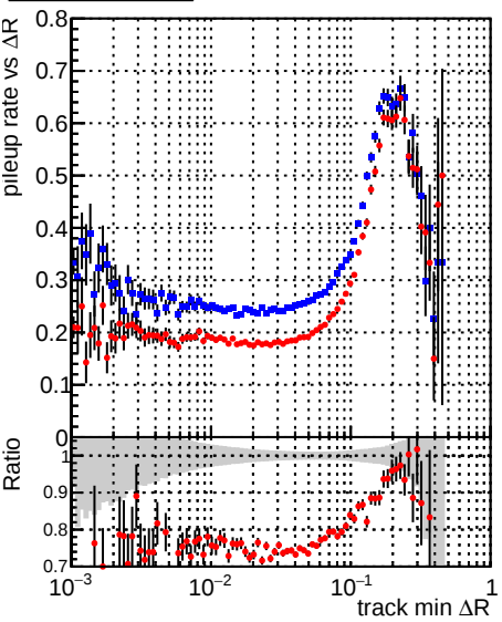
—•— DQM_mkFit_TT_base_noSel —•— DQM_mkFit_TT_retrainOldFiles_v2_8iter2_noSel
