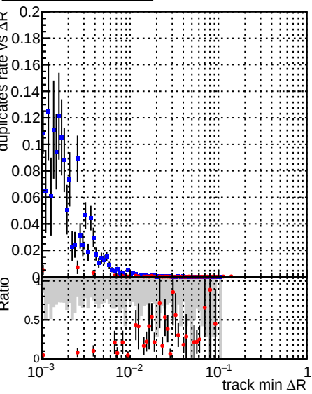
—•— DQM_mkFit_TT_base_noSel —•— DQM_mkFit_TT_retrainOldFiles_v2_8iter2_noSel
