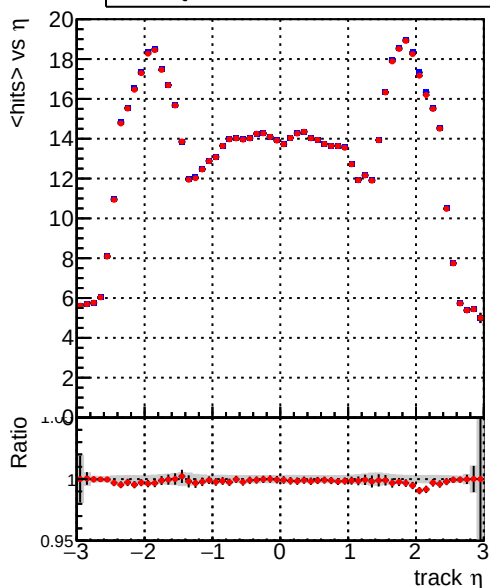
— DQM_mkFit_TT_base_noSel — DQM_mkFit_TT_retrainOldFiles_v2_8iter2_noSel
