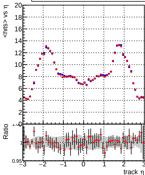
— DQM_mkFit_TT_base_noSel — DQM_mkFit_TT_retrainOldFiles_v2_8iter2_noSel mean hits
