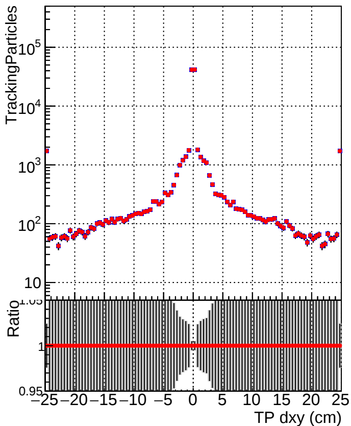
■ DQM_mkFit_TT_base_noSel ● DQM_mkFit_TT_retrainOldFiles_v2_noSel
