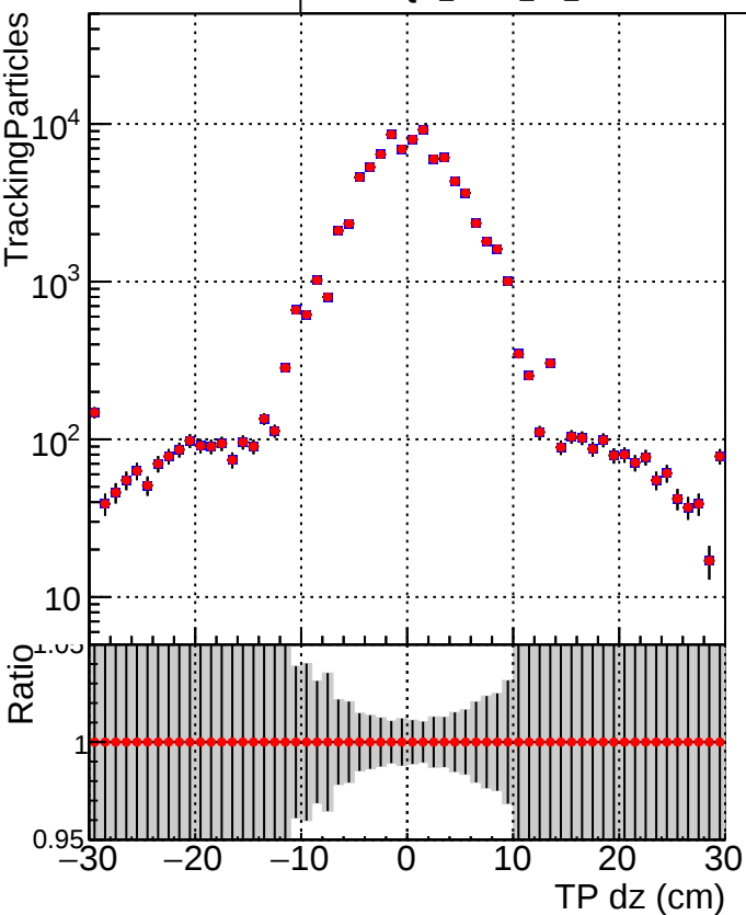
■ DQM_mkFit_TT_base_noSel ● DQM_mkFit_TT_retrainOldFiles_v2_noSel
