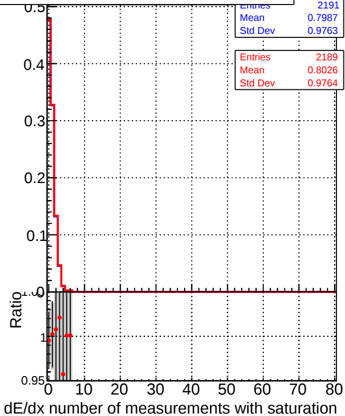
—■— DQM_mkFit_TT_base_noSel —●— DQM_mkFit_TT_retrainOldFiles_v2_noSel
