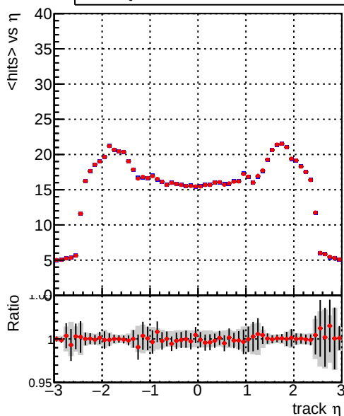
— DQM_mkFit_TT_base_noSel — DQM_mkFit_TT_retrainOldFiles_v2_noSel
