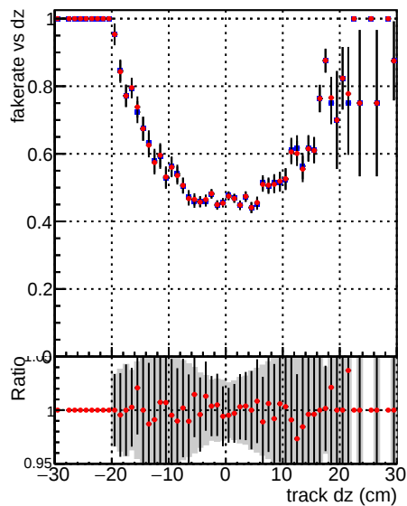
—●— DQM_mkFit_TT_base_noSel —●— DQM_mkFit_TT_retrainOldFiles_v2_noSel
