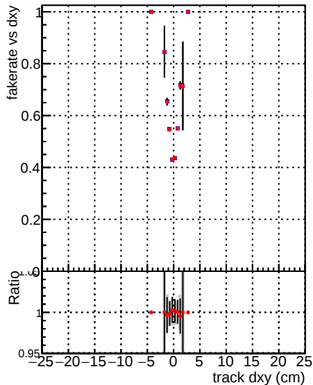
—●— DQM_mkFit_TT_base_noSel —●— DQM_mkFit_TT_retrainOldFiles_v2_noSel
