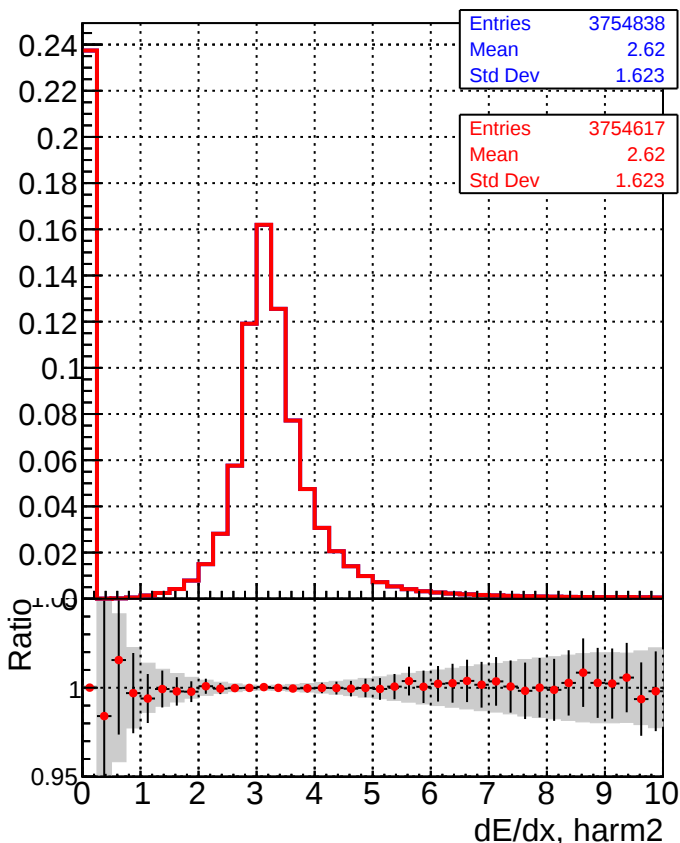
— DQM_mkFit_TT_base_noSel — DQM_mkFit_TT_retrainOldFiles_v2_noSel
