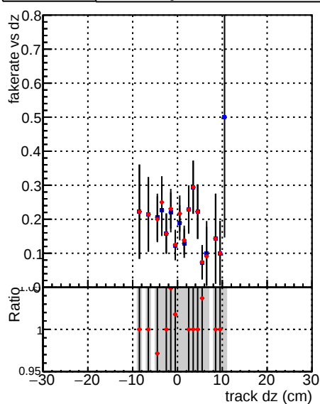
—•— DQM_mkFit_TT_base_noSel —•— DQM_mkFit_TT_retrainOldFiles_v2_noSel
