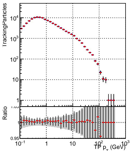
—•— DQM_mkFit_TT_base_noSel —•— DQM_mkFit_TT_retrainOldFiles_v2_noSel
