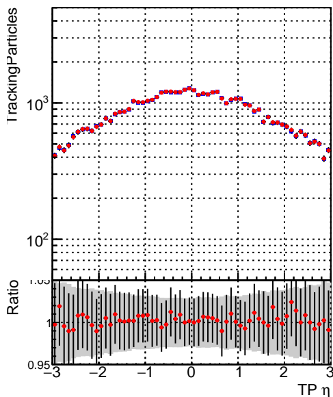
—•— DQM_mkFit_TT_base_noSel —•— DQM_mkFit_TT_retrainOldFiles_v2_noSel
