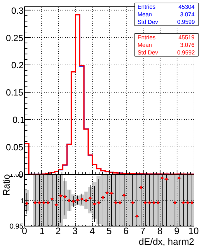
DQM_mkFit_TT_base_noSel DQM_mkFit_TT_retrainOldFiles_v2_noSel
