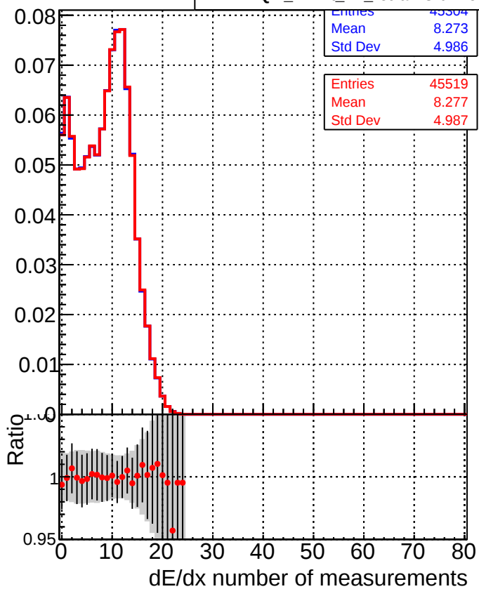
DQM_mkFit_TT_base_noSel DQM_mkFit_TT_retrainOldFiles_v2_noSel
