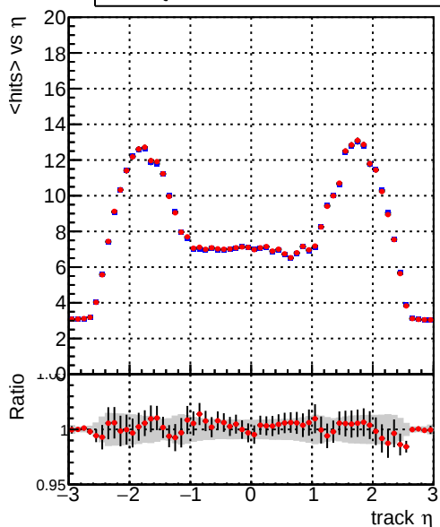
— DQM_mkFit_TT_base_noSel — DQM_mkFit_TT_retrainOldFiles_v2_noSel mean hits
