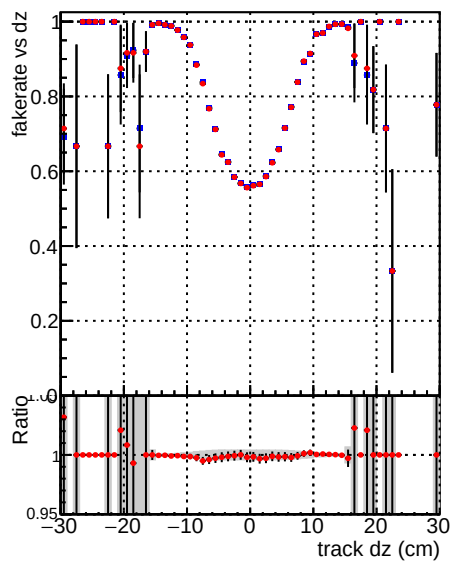
Fake rate vs dz DQM mkFit TT base_noSel DQM mkFit TT retrainOldFiles_v2_noSel
