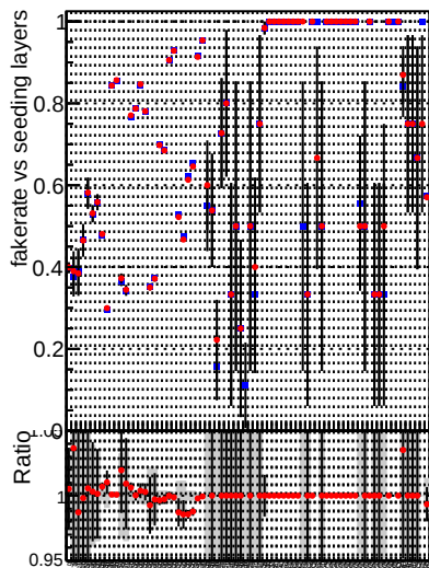
Fake rate vs. DQM mkFit TT_base_noSel DQM mkFit TT_retrainOldFiles_v2_noSel
