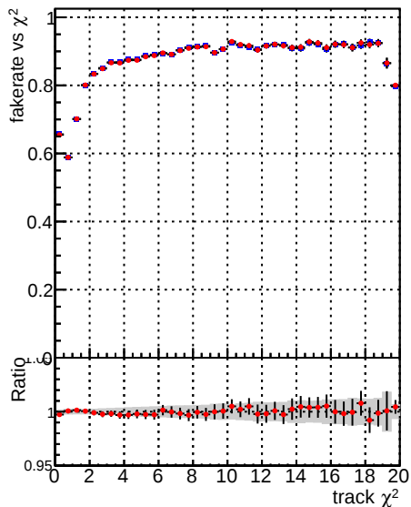
Fake rate vs. DQM mkFit TT_base_noSel DQM mkFit TT_retrainOldFiles_v2_noSel
