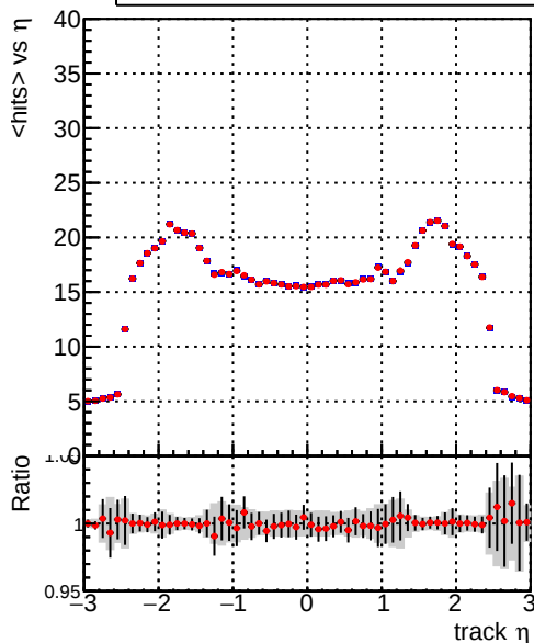
— DQM_mkFit_TT_base_noSel — DQM_mkFit_TT_retrainOldFiles_v2_noSel mean hits > \eta
