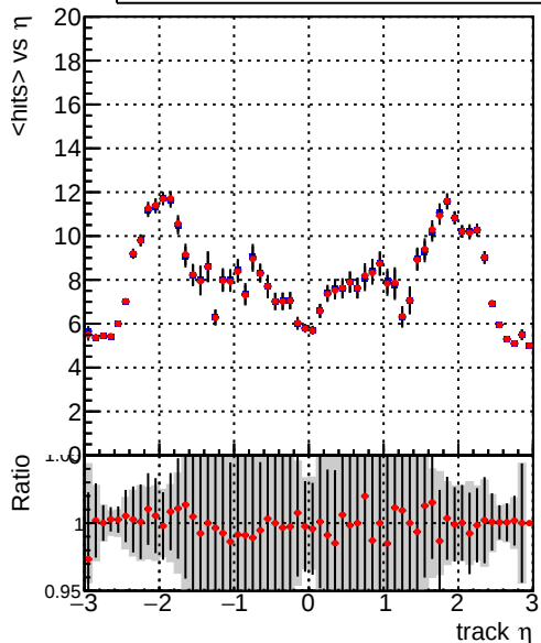
— DQM_mkFit_TT_base_noSel — DQM_mkFit_TT_retrainOldFiles_v2_noSel
