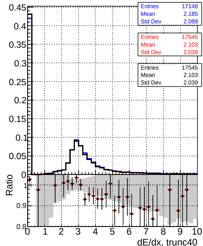
dE/dx estimator 2
