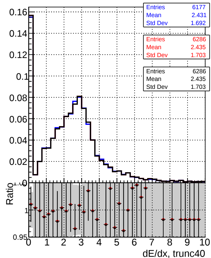
dE/dx estimator 2
