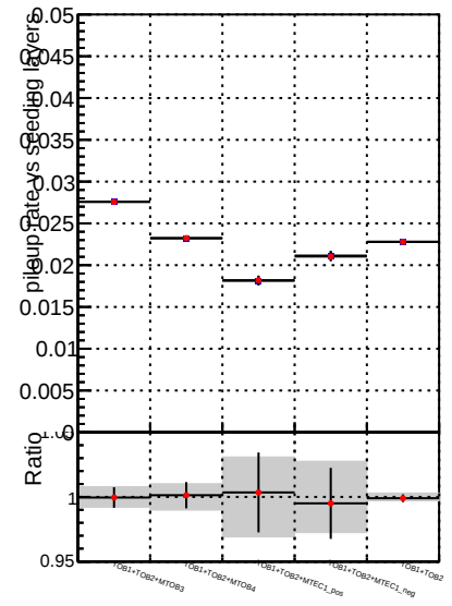
—•— DQM CKF TTbase —•— DQM CKF TT_retrainOldFiles125_v2_prelimWP3_epoch4
