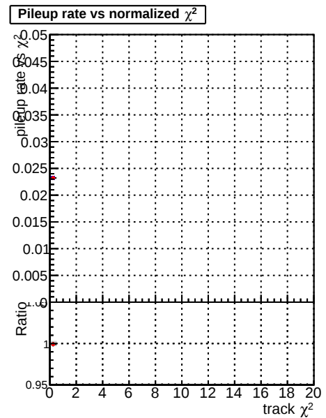
—•— DQM CKF TTbase —•— DQM CKF TT_retrainOldFiles125_v2_prelimWP3_epoch4
