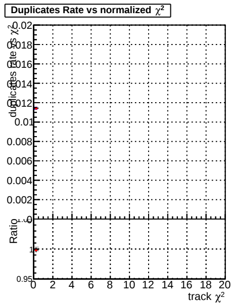
—•— DQM CKF TTbase —•— DQM CKF TT_retrainOldFiles125_v2_prelimWP3_epoch4
