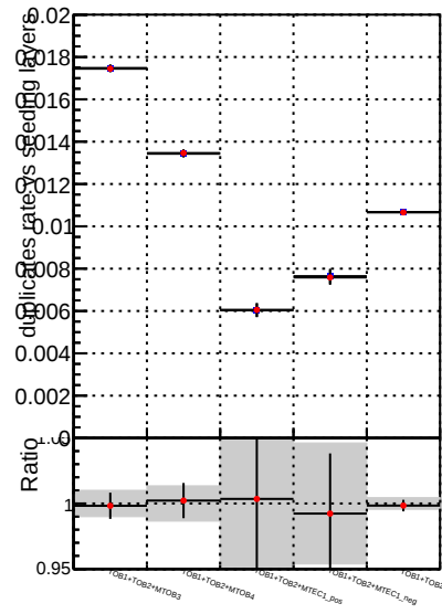
—•— DQM CKF TTbase —•— DQM CKF TT_retrainOldFiles125_v2_prelimWP3_epoch4
