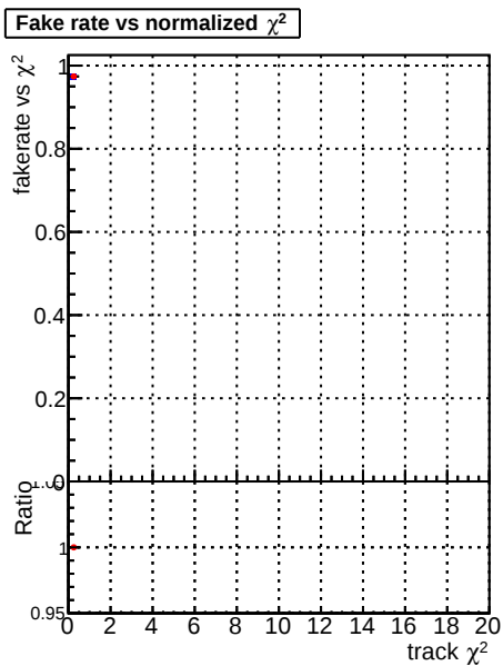
—•— DQM CKF TTbase —•— DQM CKF TT_retrainOldFiles125_v2_prelimWP3_epoch4
