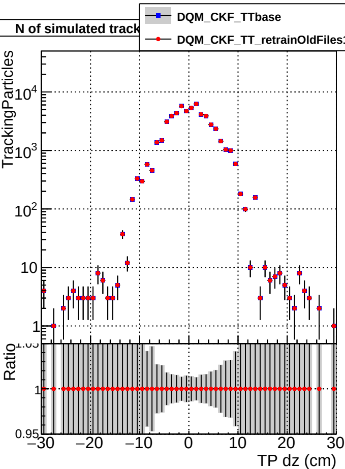
■ DQM_CKF_TTbase ■ DQM_CKF_TT_retrainOldFiles125_v2_prelimWP3_epoch4
