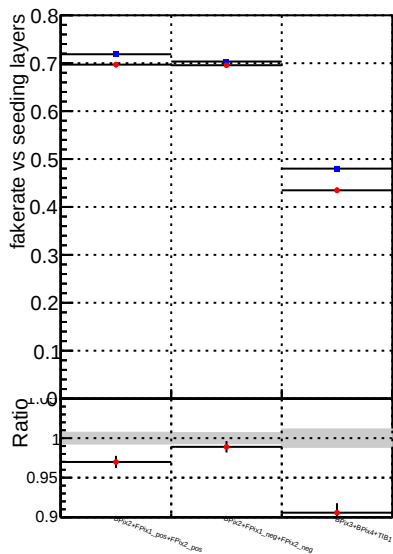
Fake rate vs. —•— DQM CKF TTbase —•— DQM CKF TT_retrainOldFiles125_v2_prelimWP3_epoch4
