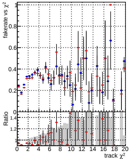
Fake rate vs. \chi^2 Legend: —•— DQM CKF TTbase —•— DQM CKF TT_retrainOldFiles125_v2_prelimWP3_epoch4
