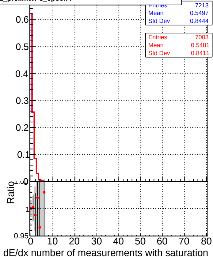
DQM_CKF_TTbase DQM_CKF_TT_retrainOldFiles125_v2_prelimWP3_epoch4
