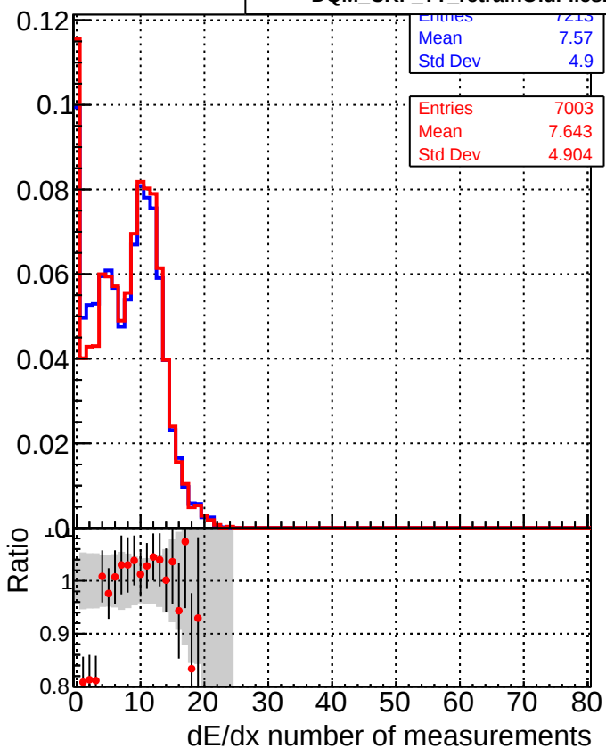
DQM_CKF_TTbase DQM_CKF_TT_retrainOldFiles125_v2_prelimWP3_epoch4
