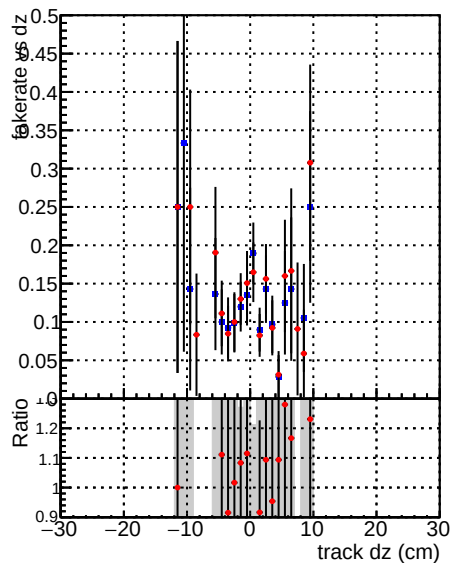
—●— DQM CKF TTbase —●— DQM CKF TT_retrainOldFiles125_v2_prelimWP3_epoch4
