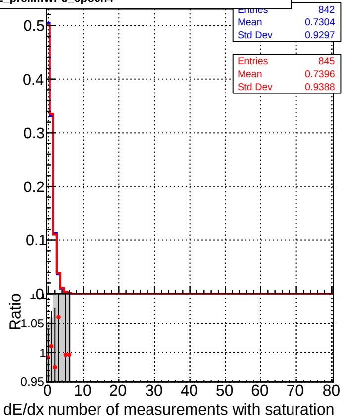
DQM_CKF_TTbase DQM_CKF_TT_retrainOldFiles125_v2_prelimWP3_epoch4
