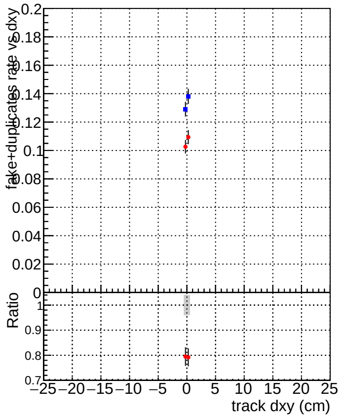
DQM_CKF_TTbase DQM_CKF_TT_retrainOldFiles125_v2_prelimWP3_epoch4
