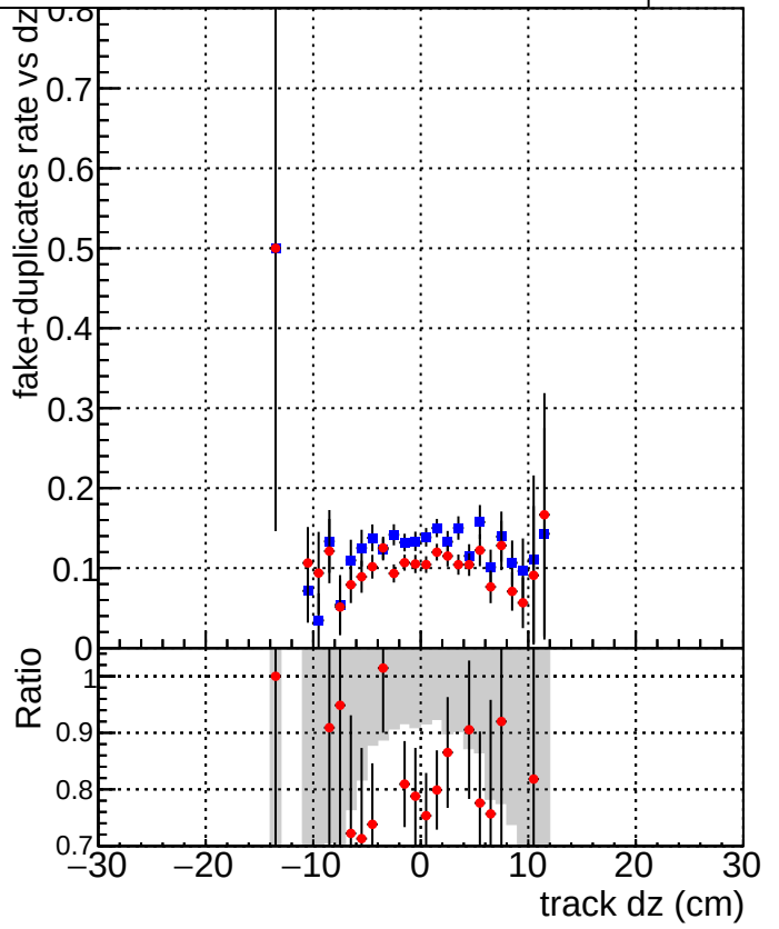
DQM_CKF_TTbase DQM_CKF_TT_retrainOldFiles125_v2_prelimWP3_epoch4
