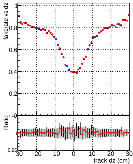
—●— DQM CKF TTbase —●— DQM CKF TT_retrainOldFiles125_v2_prelimWP3_epoch4 Fake rate vs dz
