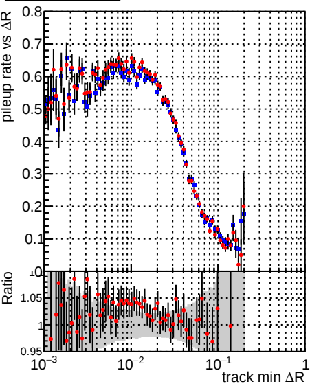
DQM_CKF_TTbase DQM_CKF_TT_retrainOldFiles125_v2_prelimWP2_epoch4
