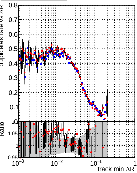
DQM_CKF_TTbase DQM_CKF_TT_retrainOldFiles125_v2_prelimWP2_epoch4
