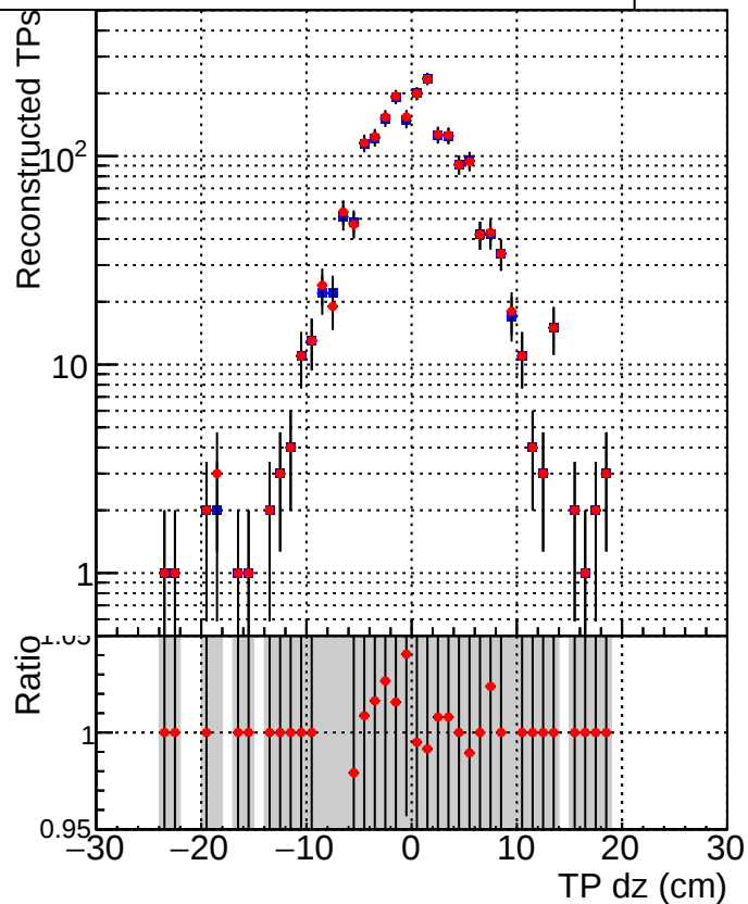
DQM_CKF_TTbase DQM_CKF_TT_retrainOldFiles125_v2_prelimWP2_epoch4
