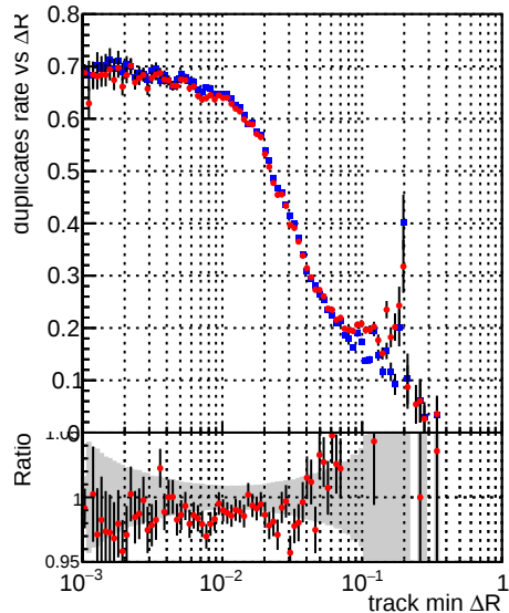
— DQM_CKF_TTbase — DQM_CKF_TT_retrainOldFiles125_v2_prelimWP2_epoch4
