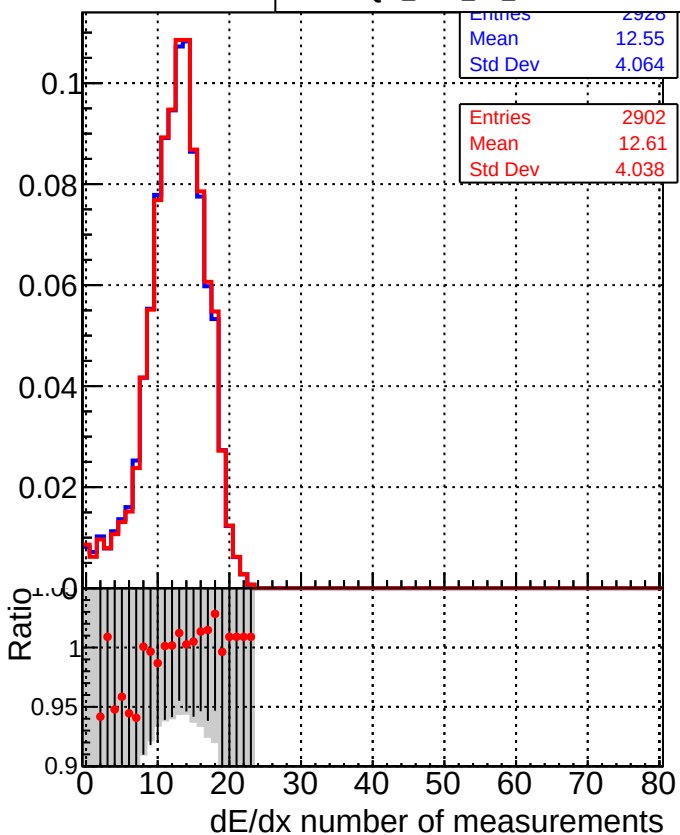
■ DQM_CKF_TTbase ● DQM_CKF_TT_retrainOldFiles125_v2_prelimWP2_epoch4
