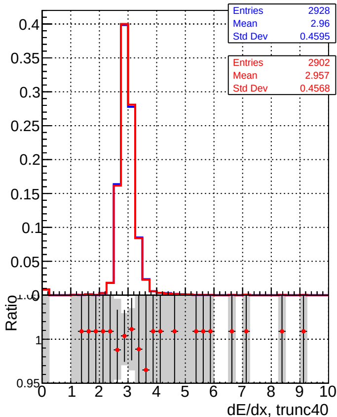
■ DQM_CKF_TTbase ● DQM_CKF_TT_retrainOldFiles125_v2_prelimWP2_epoch4
