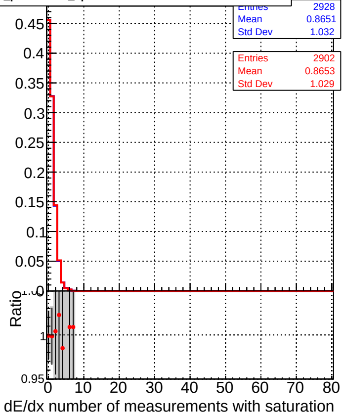
■ DQM_CKF_TTbase ● DQM_CKF_TT_retrainOldFiles125_v2_prelimWP2_epoch4
