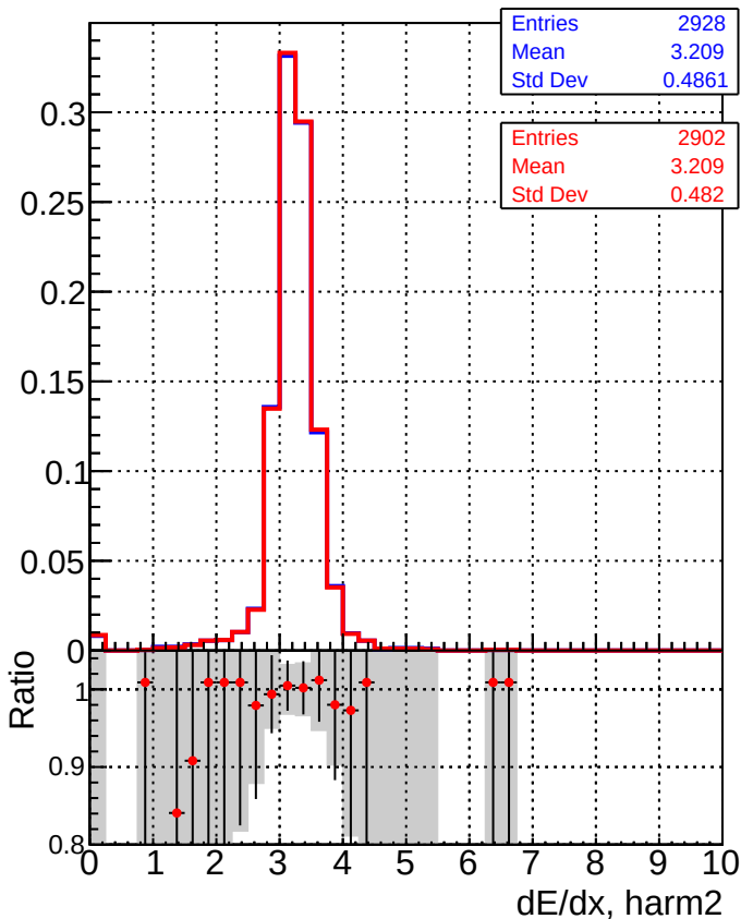
■ DQM_CKF_TTbase ● DQM_CKF_TT_retrainOldFiles125_v2_prelimWP2_epoch4
