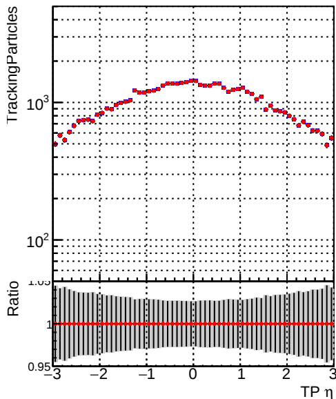
■ DQM_CKF_TTbase —●— DQM_CKF_TT_retrainOldFiles125_v2_prelimWP2_epoch4
