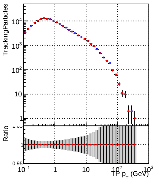
■ DQM_CKF_TTbase —●— DQM_CKF_TT_retrainOldFiles125_v2_prelimWP2_epoch4
