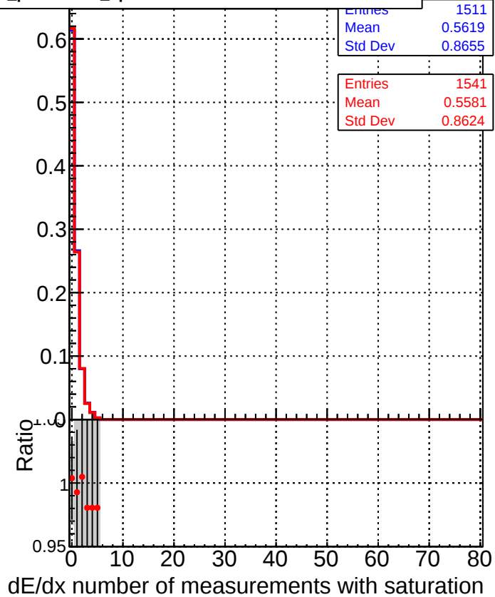
■ DQM_CKF_TTbase ● DQM_CKF_TT_retrainOldFiles125_v2_prelimWP2_epoch4
