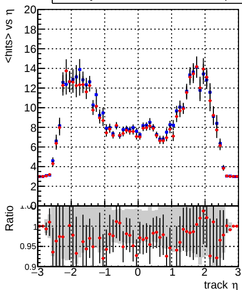
— DQM_CKF_TTbase — DQM_CKF_TT_retrainOldFiles125_v2_prelimWP2_epoch4
