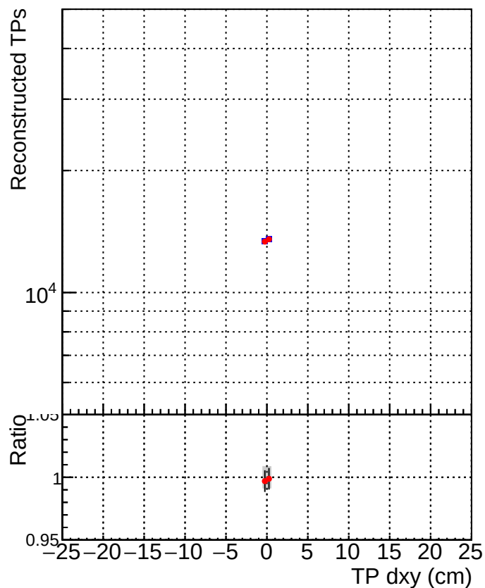
■ DQM_CKF_TTbase ■ DQM_CKF_TT_retrainOldFiles125_v2_prelimWP2_epoch4
