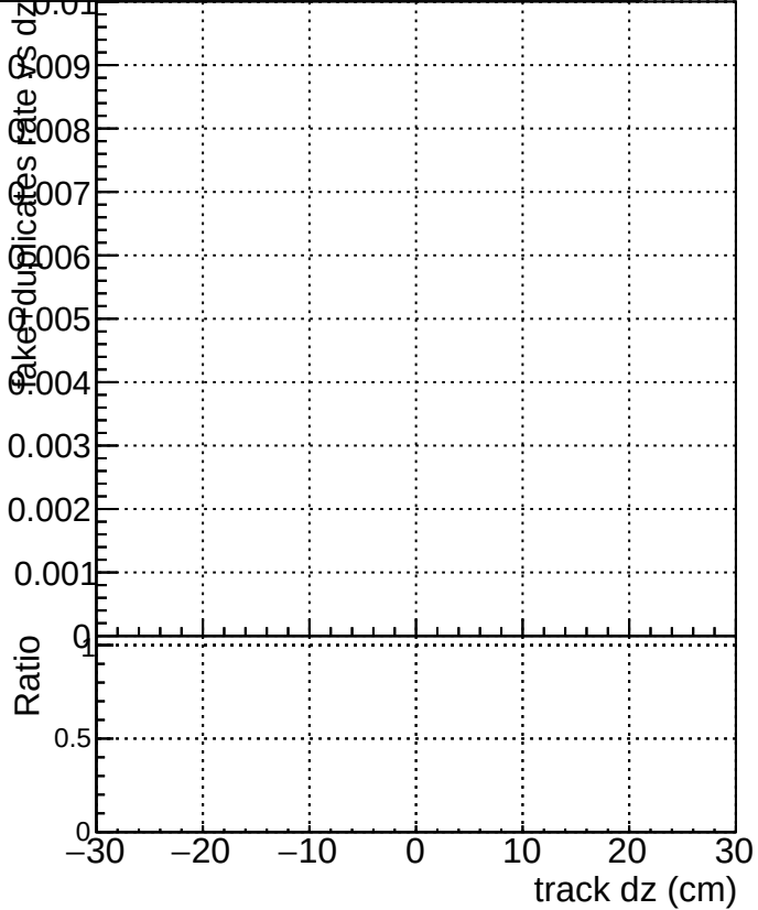
DQM_CKF_TTbase DQM_CKF_TT_retrainOldFiles125_v2_prelimWP2_epoch4
