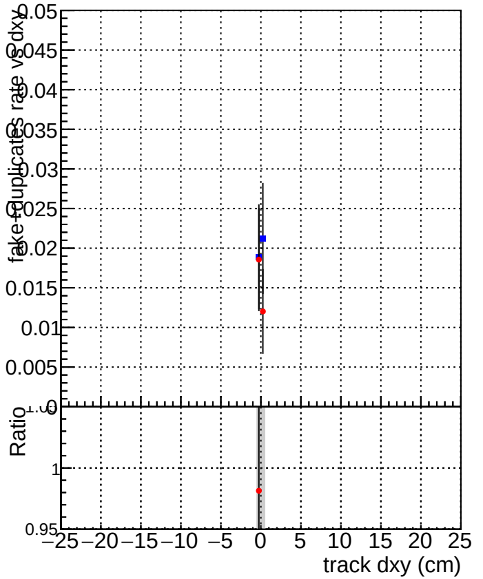
DQM_CKF_TTbase DQM_CKF_TT_retrainOldFiles125_v2_prelimWP2_epoch4
