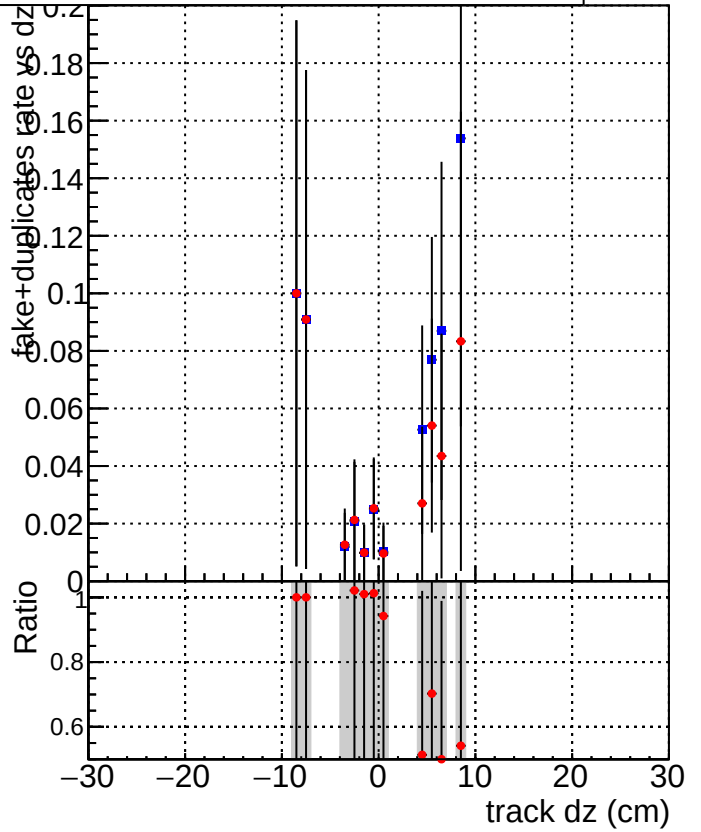
DQM_CKF_TTbase DQM_CKF_TT_retrainOldFiles125_v2_prelimWP2_epoch4
