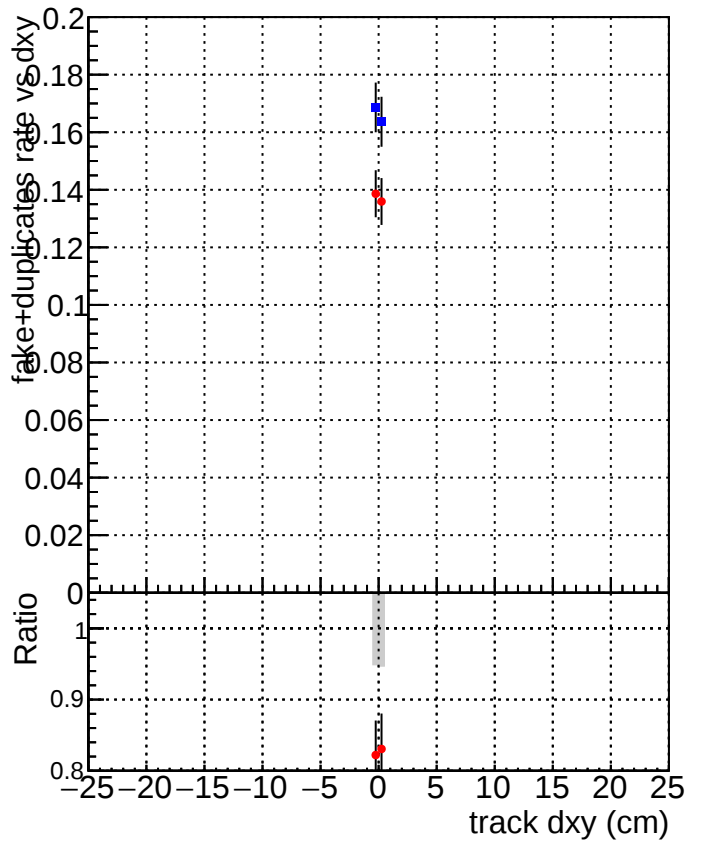
DQM_CKF_TTbase DQM_CKF_TT_retrainOldFiles125_v2_prelimWP2_epoch4
