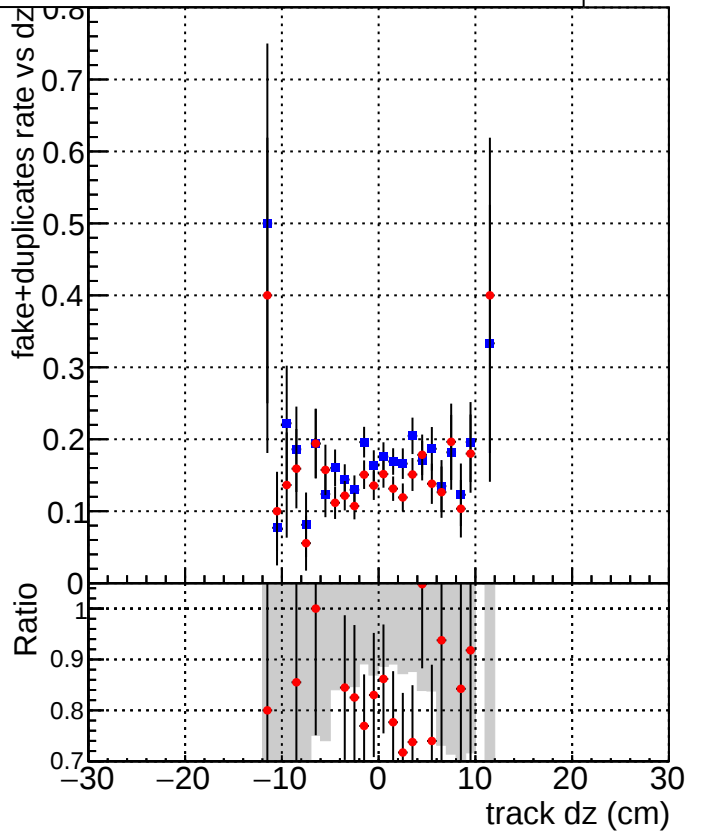
DQM_CKF_TTbase DQM_CKF_TT_retrainOldFiles125_v2_prelimWP2_epoch4
