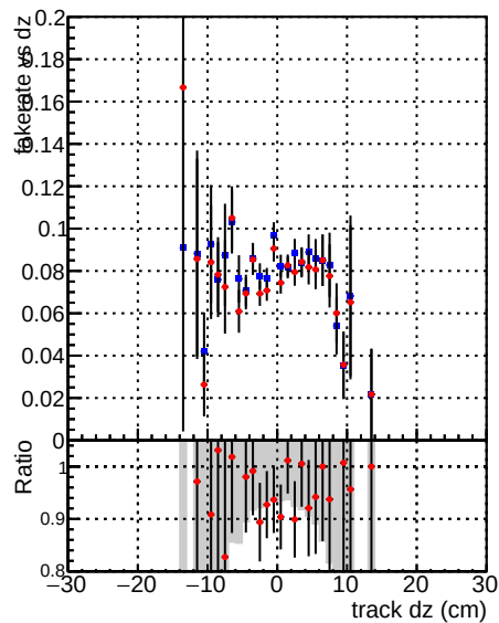
—●— DQM CKF TTbase —●— DQM CKF TT_retrainOldFiles125_v2_prelimWP2_epoch4
