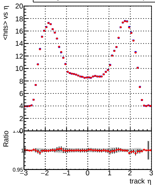
— DQM_CKF_TTbase — DQM_CKF_TT_retrainOldFiles125_v2_prelimWP2_epoch4
