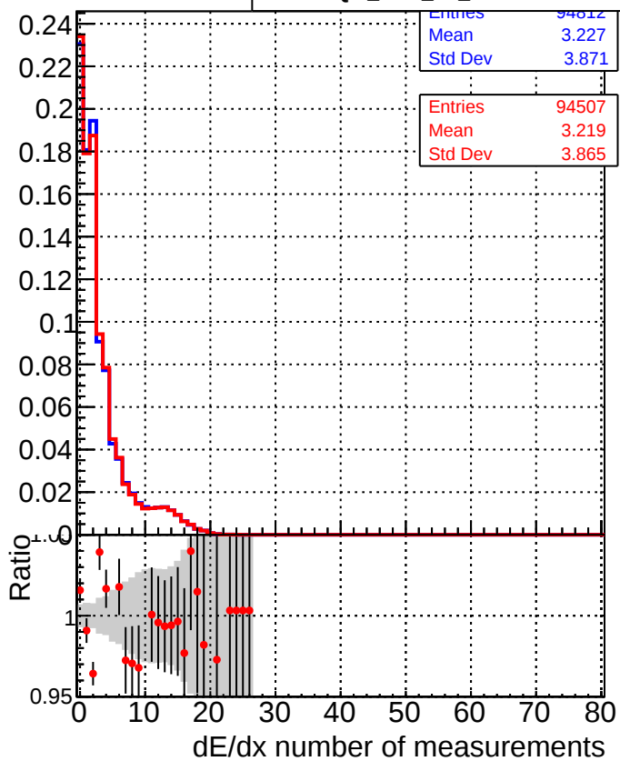
■ DQM_CKF_TTbase ● DQM_CKF_TT_retrainOldFiles125_v2_prelimWP2_epoch4
