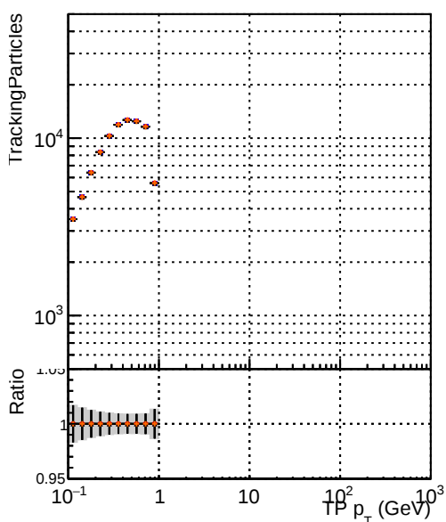
—●— DQM_mkFit_TTbase —●— DQM_mkFit_TT_retrainOldFiles125_v2_prelimWP_5iter —●— DQM_mkFit_TT_baseline_6iter —●— DQM_mkFit_TT_RetrainV2_WP2_6iter
