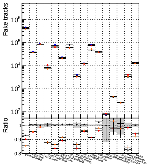
Number Series 1 DQM_mkFit_TT_retrainOldFiles125_V2_prelimWP_5iter 2 DQM_mkFit_TT_baseline_6iter 3 DQM_mkFit_TT_RetrainV2_WP2_6iter
