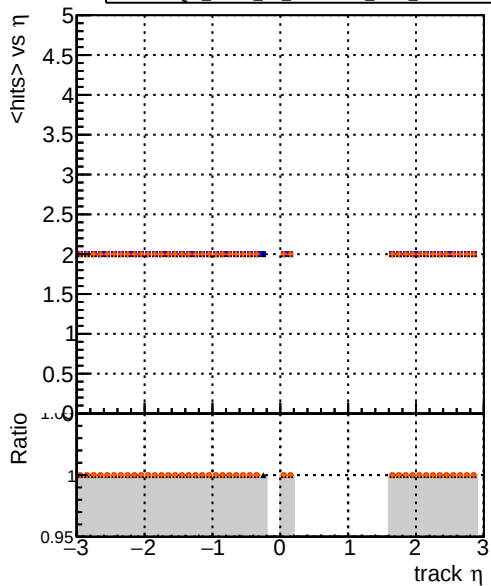
— DQM_mkFit_TTbase — DQM_mkFit_TT_retrainOldFiles125_v2_prelimWP_5iter — DQM_mkFit_TT_baseline_6iter — DQM_mkFit_TT_RetrainV2_WP2_6iter
