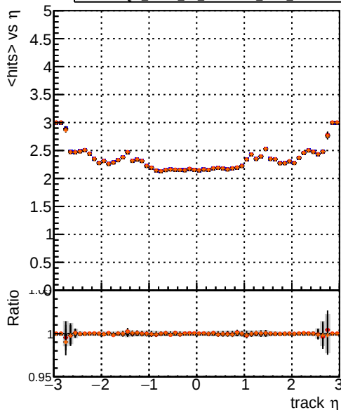
mean hits vs \eta DQM_mkFit_TTbase DQM_mkFit_TT_retrainOldFiles125_v2_prelimWP_5iter DQM_mkFit_TT_baseline_6iter DQM_mkFit_TT_RetrainV2_WP2_6iter
