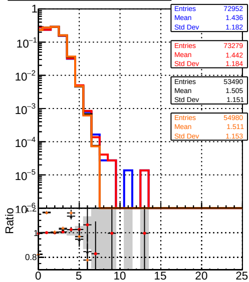
Legend: — DQM_mkFit_TTbase — DQM_mkFit_TT_retrainOldFiles125_v2_prelimWP_5iter — DQM_mkFit_TT_baseline_6iter — DQM_mkFit_TT_RetrainV2_WP2_6iter
