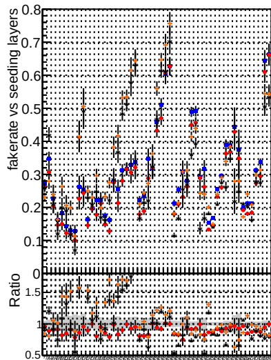
Fake rate vs. ● DQM mkFit Tbase × Data OldFiles125 v2 prelimWP_5iter × DQM mkFit Tbase × Data OldFiles125 v2 prelimWP_5iter
