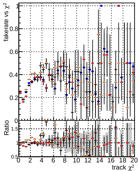
Fake rate vs. ● DQM mkFit Tbase × Data OldFiles125 v2 prelimWP_5iter × DQM mkFit Tbase × Data OldFiles125 v2 prelimWP_5iter
