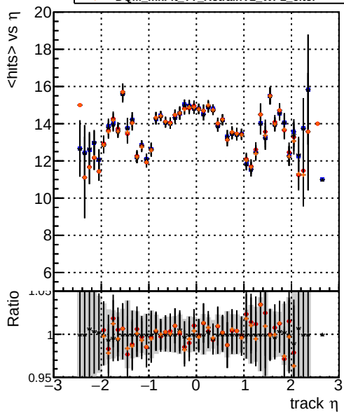
mean hit DQM_mkFit_TTbase DQM_mkFit_TT_retrainOldFiles125_v2_prelimWP_5iter DQM_mkFit_TT_baseline_6iter DQM_mkFit_TT_RetrainV2_WP2_6iter
